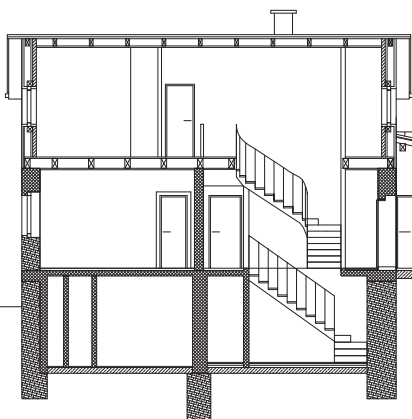
PREREZ A-A
