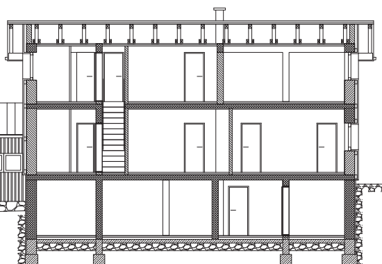
VZDOLŽNA PREREZA , M 1:100
