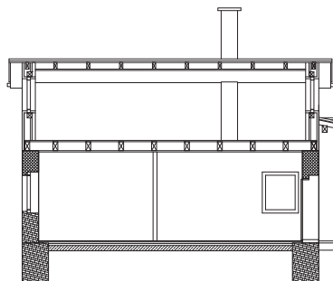
PREREZ A-A
